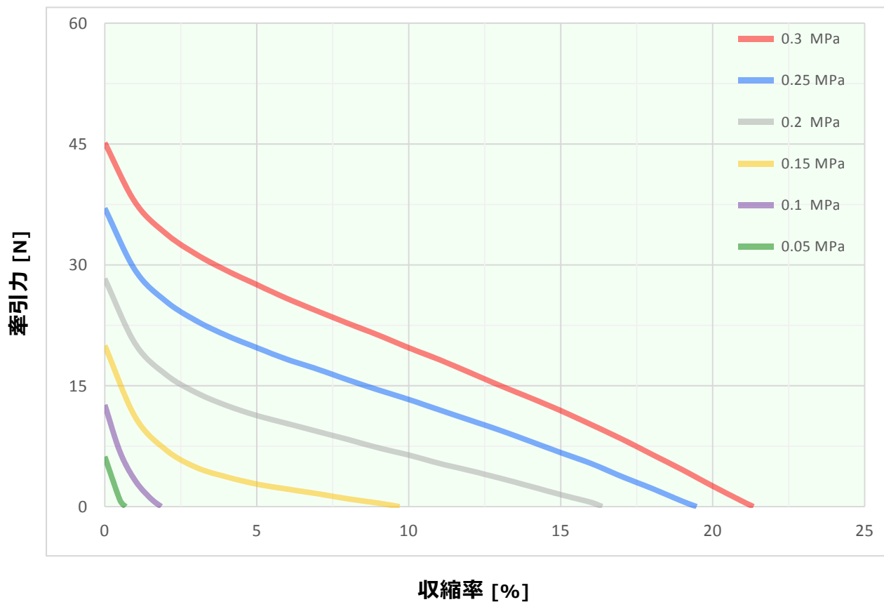
【PMJ40シリーズ】 牽引力と収縮率の関係 (参考資料)
