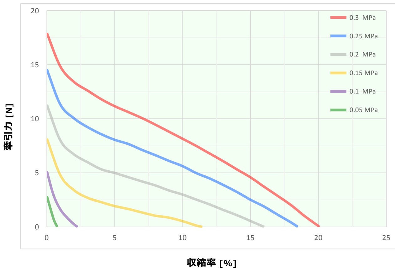
【PMJ20シリーズ】 牽引力と収縮率の関係 (参考資料)
